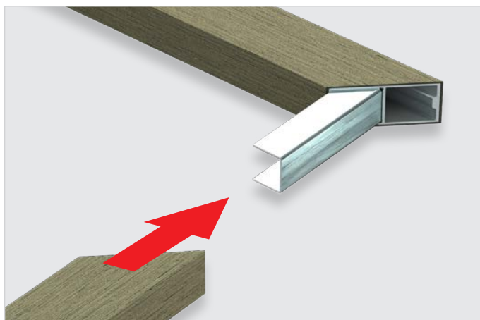
Insert profile.
